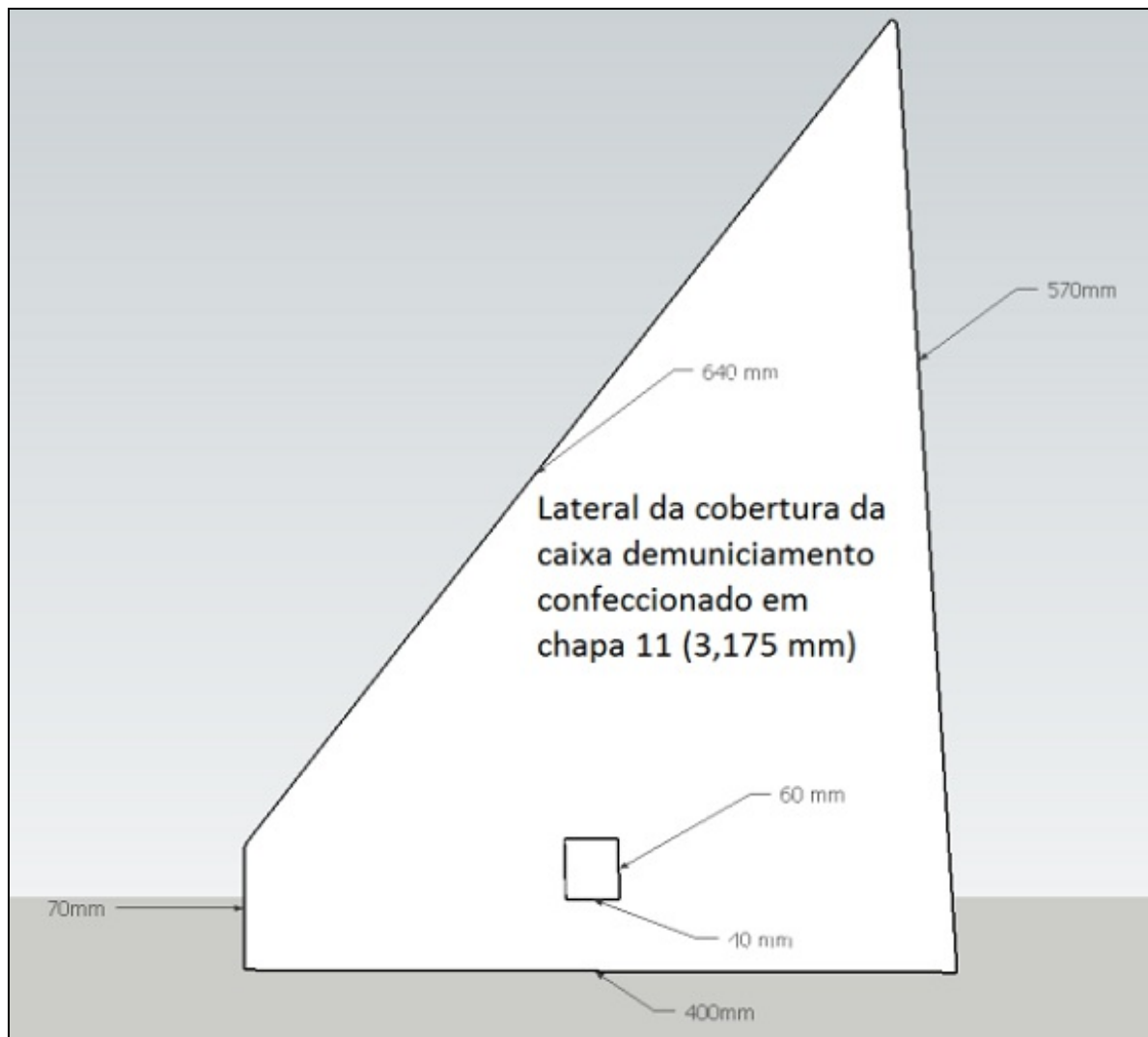
Figura 6 - Vista lateral da tampa defletora.
