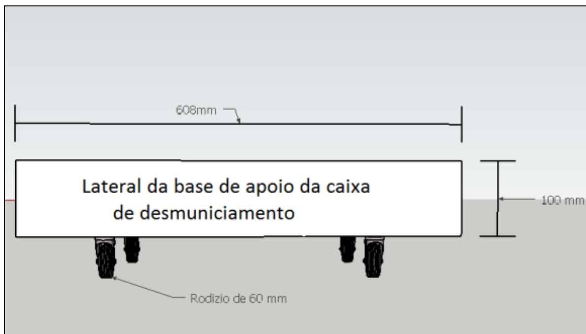
Figura 4 - Vista frontal do suporte.
