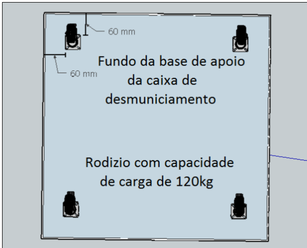
Figura 5 - Vista do fundo do suporte.
