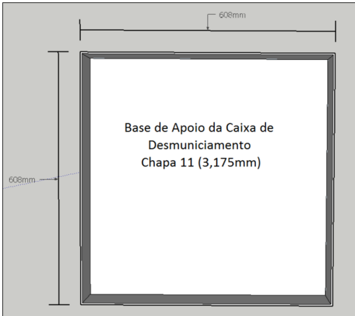
Figura 3 - Vista superior do suporte.
