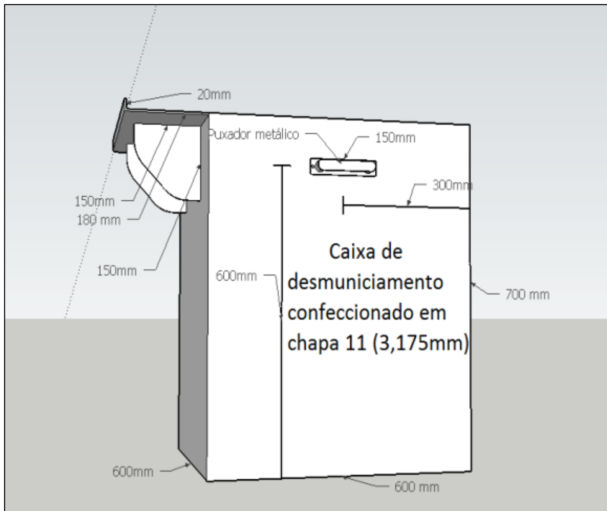
Figura 1 - Vista lateral da caixa.
